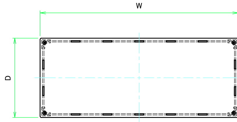
上カバー / Top cover
